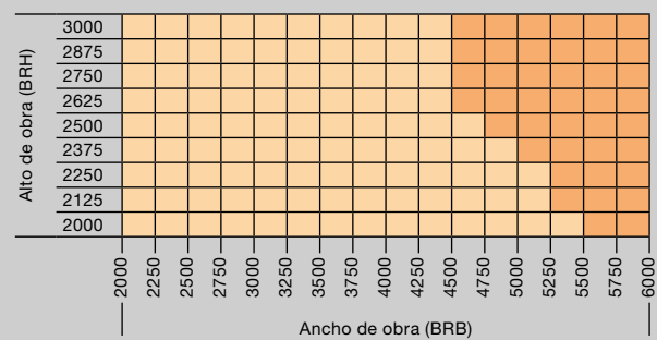
Modelo 470 NOVEDAD Revestimiento con varillas de aluminio 20 x 20 x 2 mm
