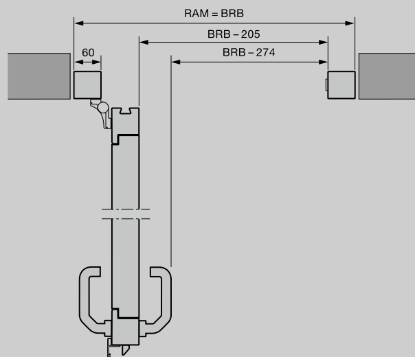
Ancho de paso libre con un ángulo de apertura de 90°
